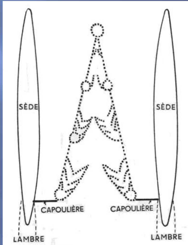
Dessin de principe d'une bourdigue
